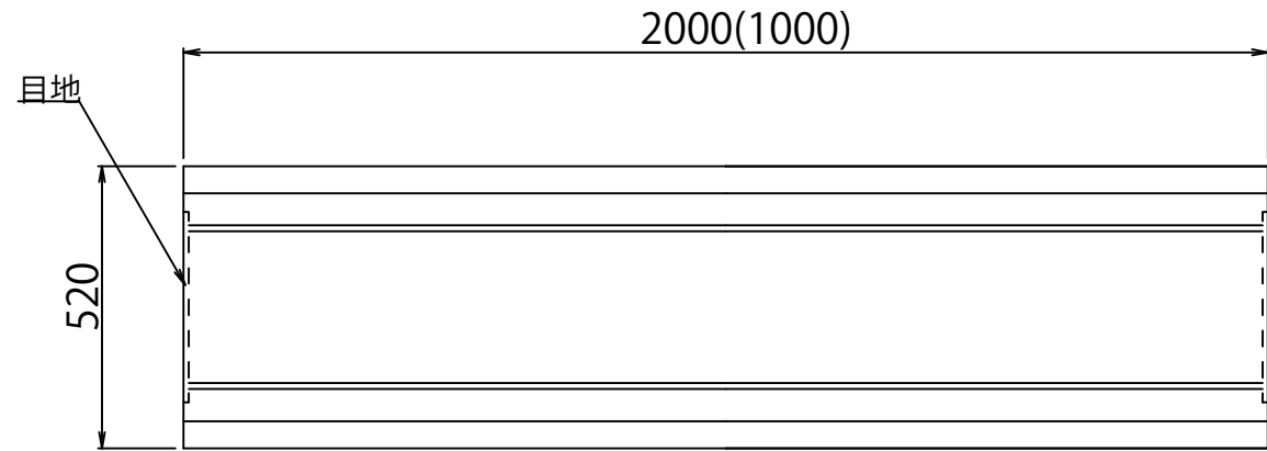
平面図
