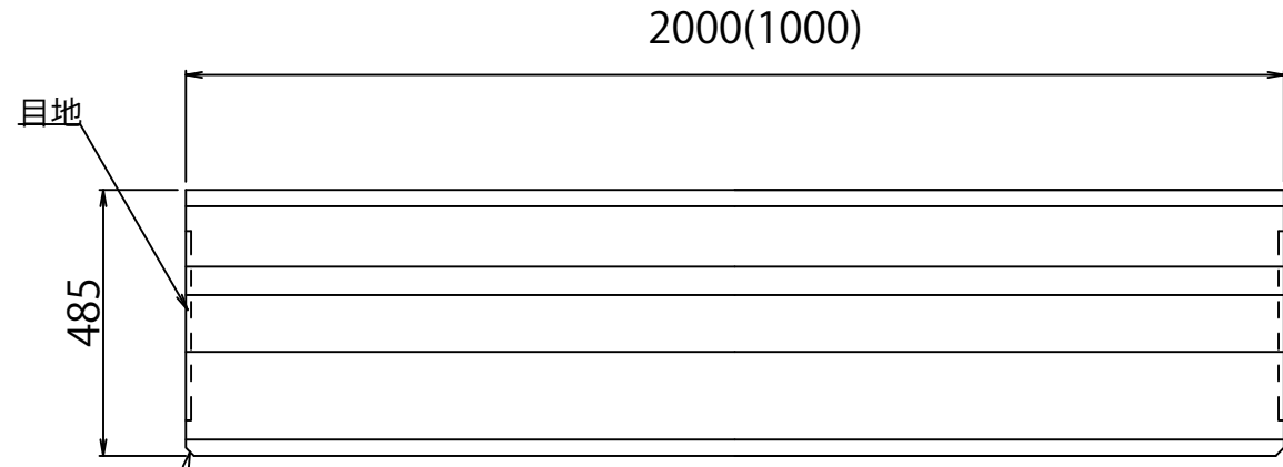
側面図
