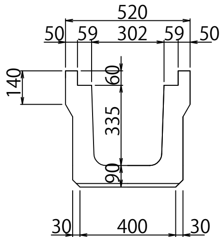
正面図
