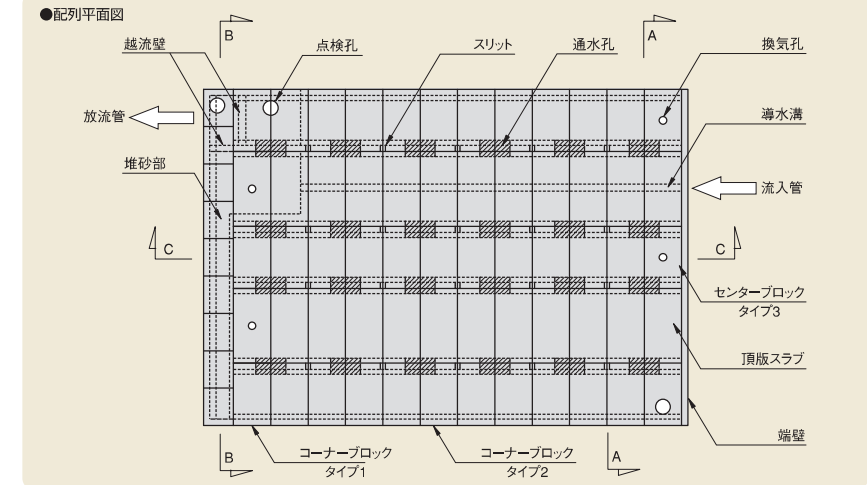
■ボックス型タイプ施設図例
